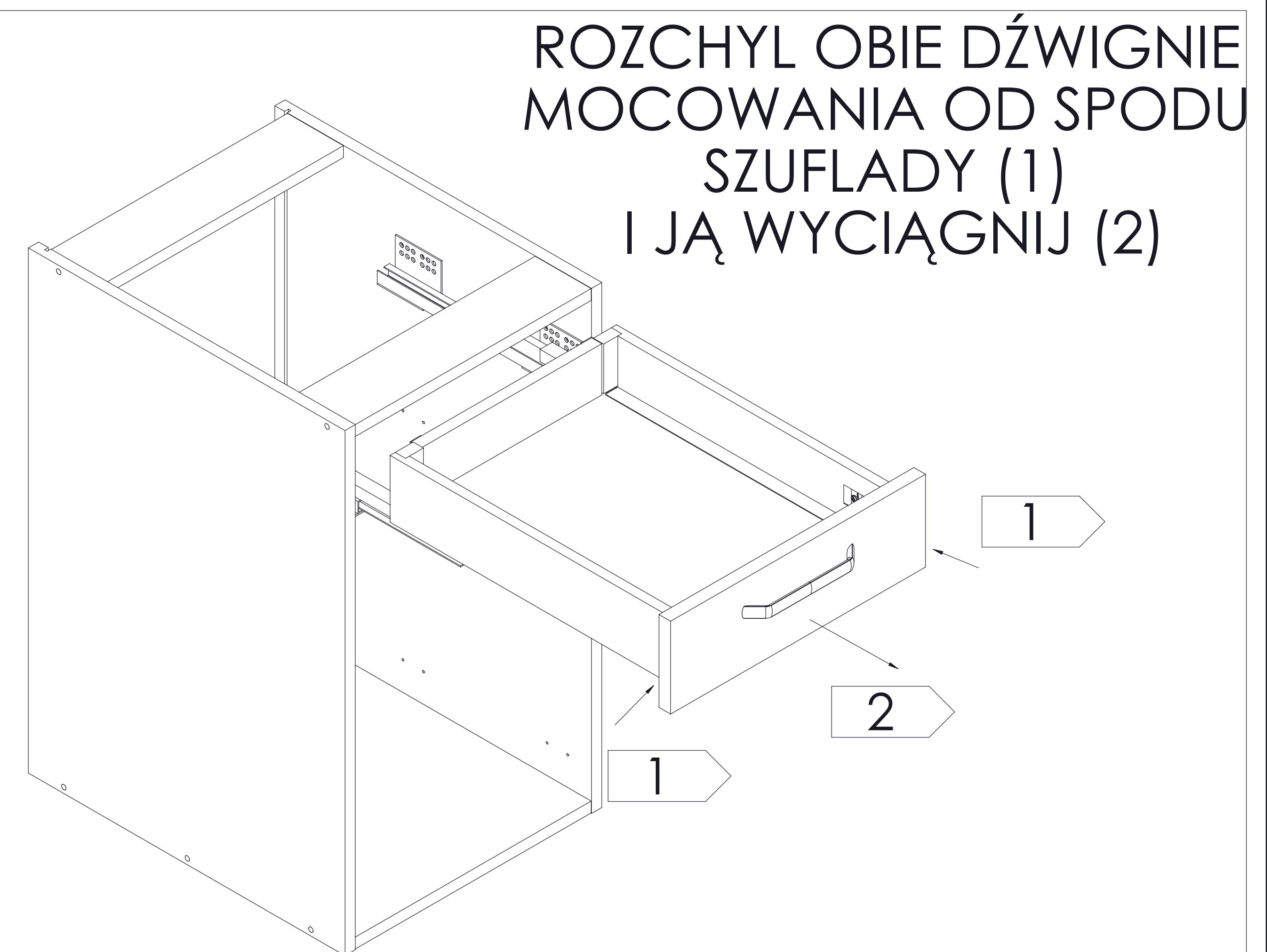
DEMONTAŻ SZUFLADY
