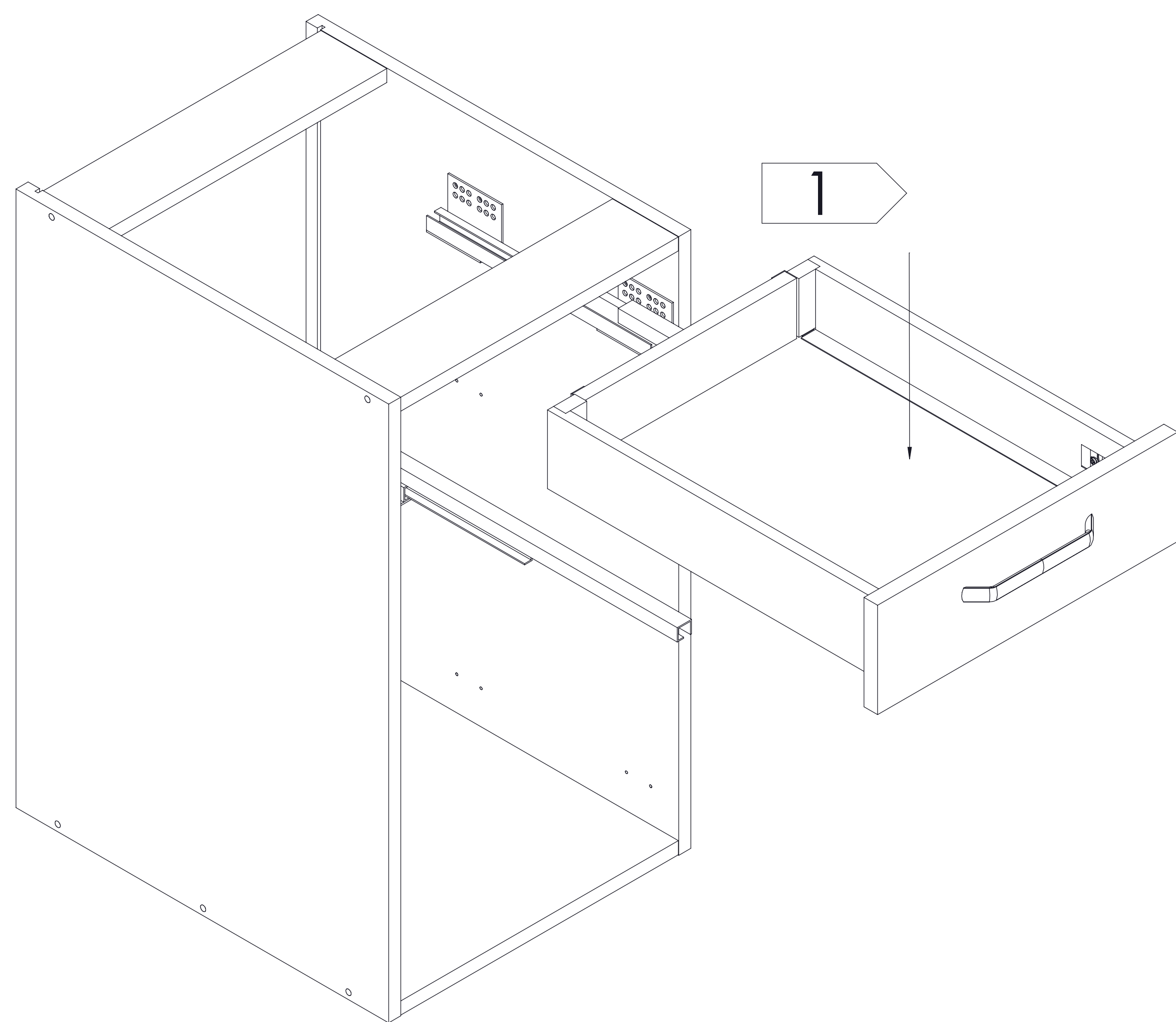
MONTAŻ SZUFLADY
